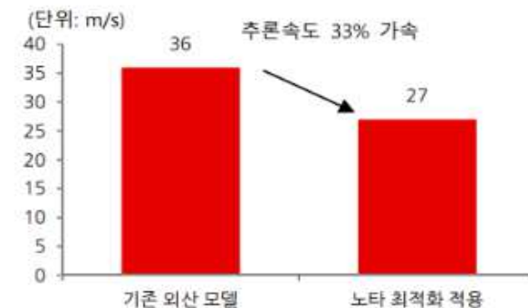
Fig. 8: Arm NPU에 노타 적용 후 속도 차이
